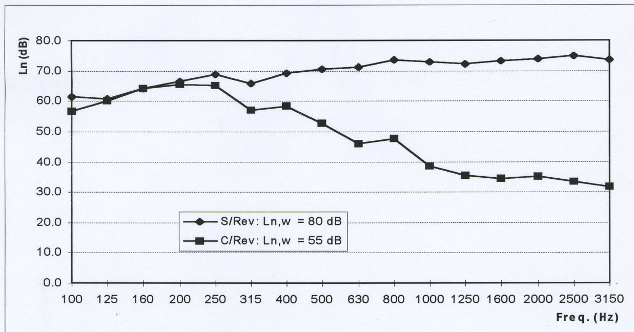
Curvas características da transmissão de sons de percussão
